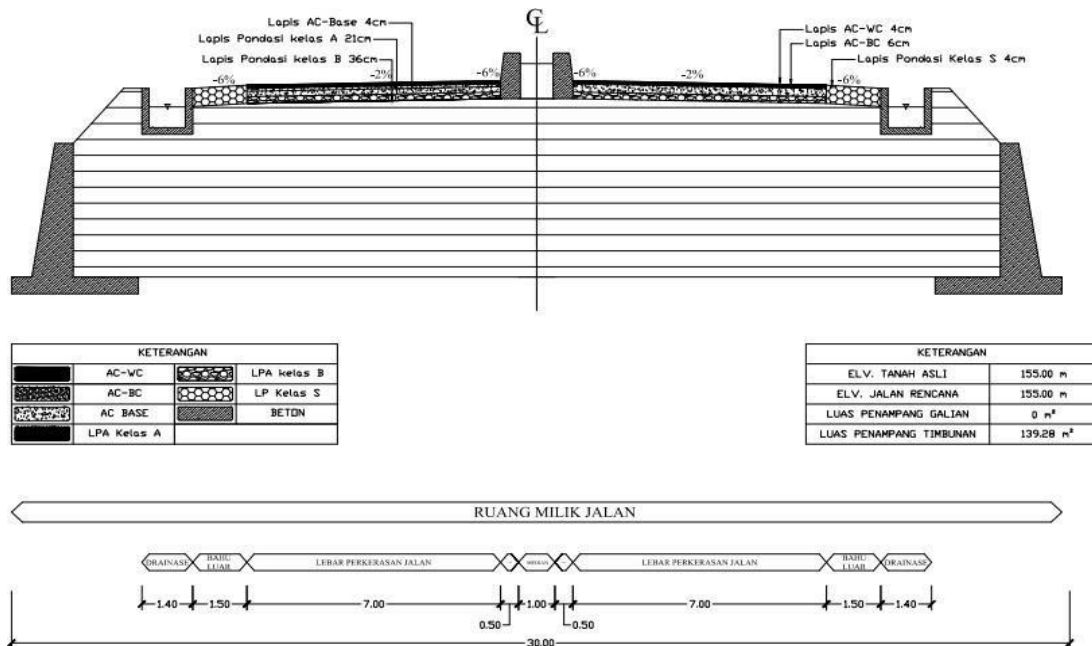
Gambar 1. Potongan Melintang Jalan
